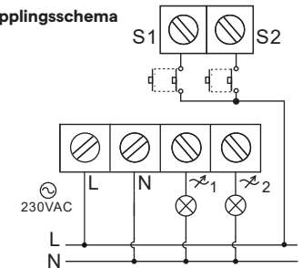
Kopplingschema
